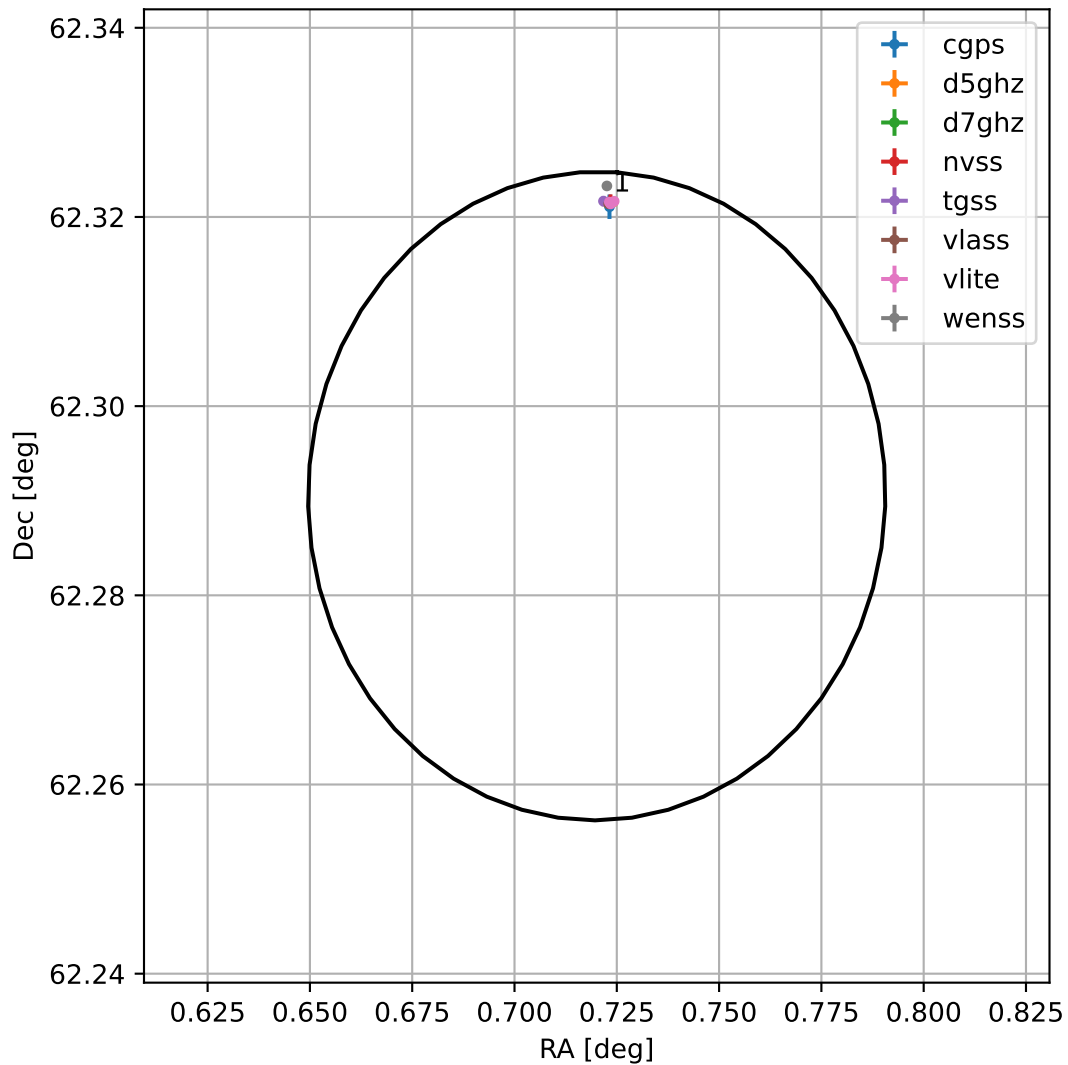
4FGL J0002.8+6217
