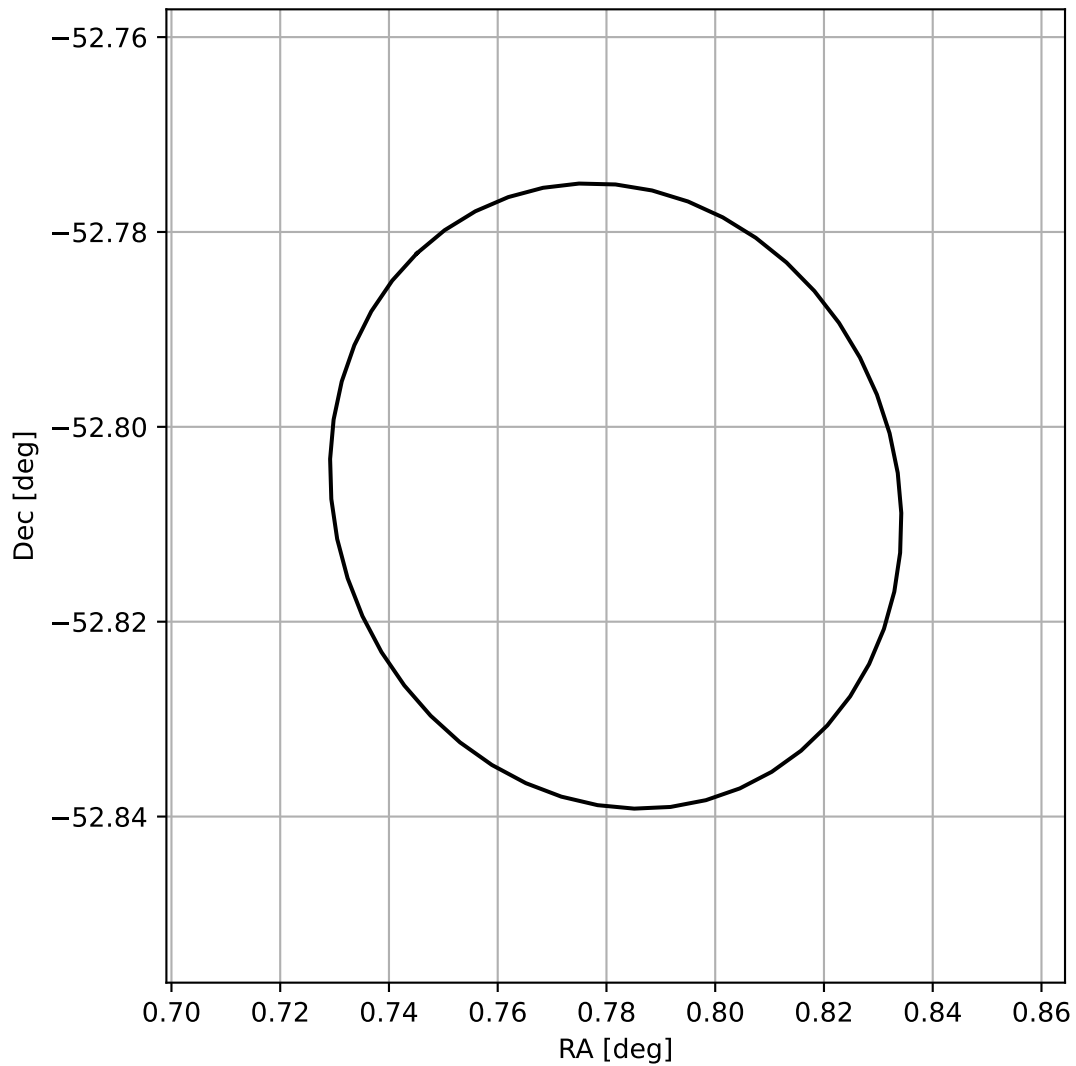
4FGL J0003.1-5248
