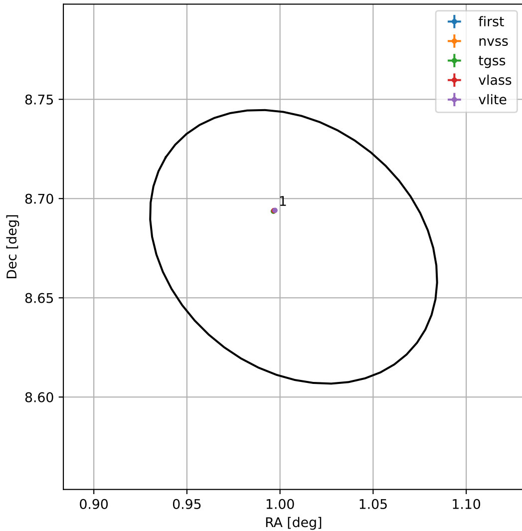
4FGL J0004.0+0840
