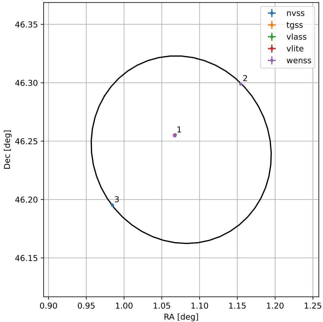
4FGL J0004.3+4614
