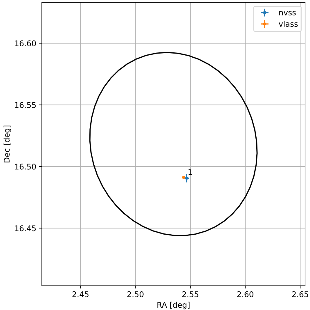
4FGL J0010.1+1631
