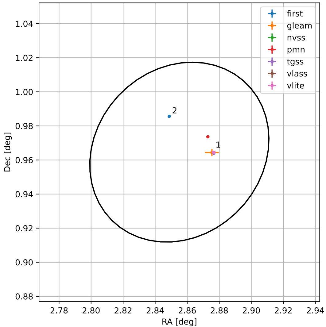
4FGL J0011.4+0057
