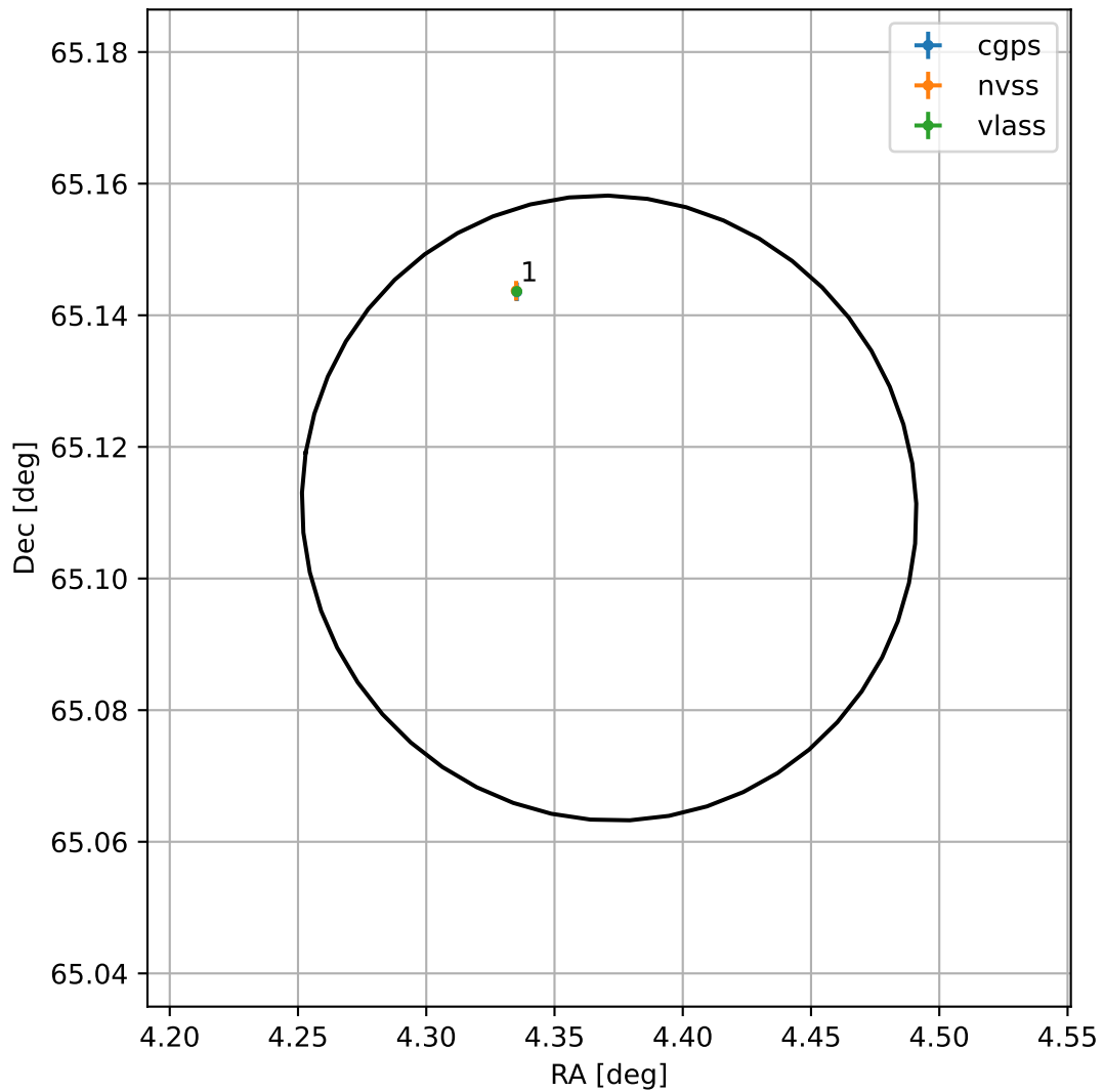
4FGL J0017.4+6506
