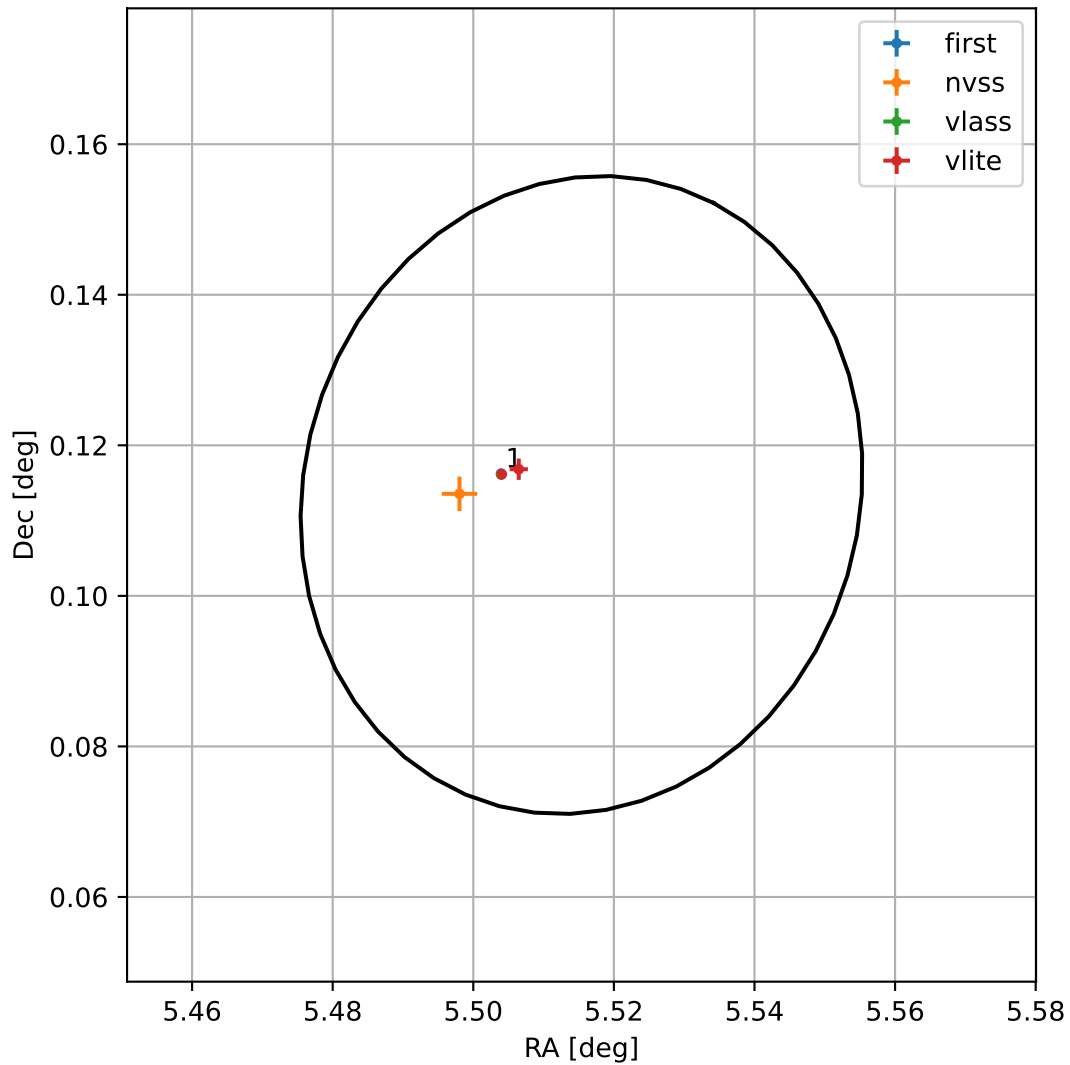
4FGL J0022.0+0006
