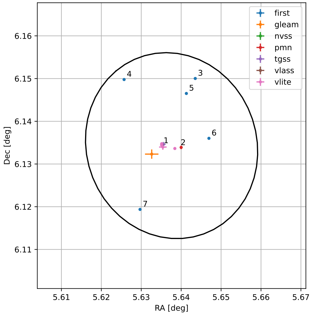
4FGL J0022.5+0608
