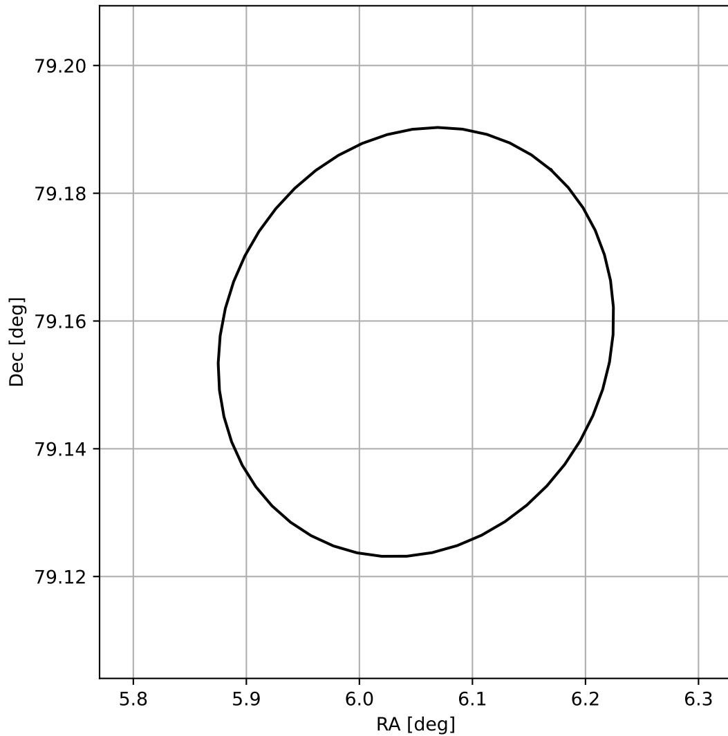
4FGL J0024.1+7909
