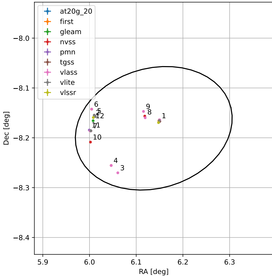
4FGL J0024.5-0810
