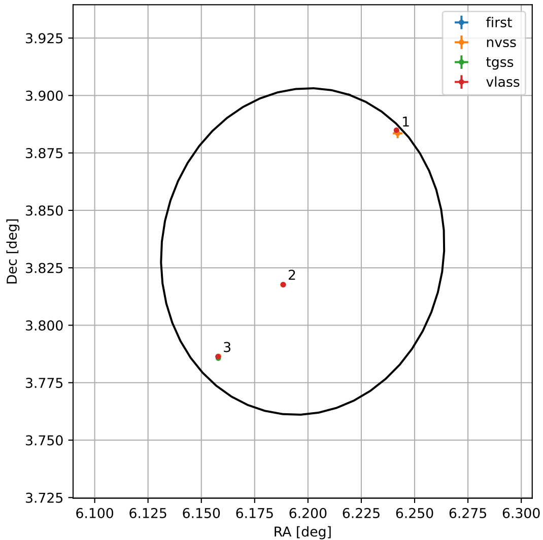
4FGL J0024.7+0349
