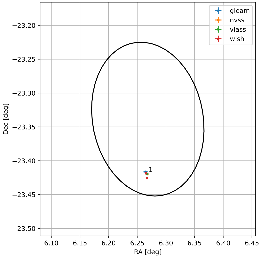
4FGL J0025.0-2320
