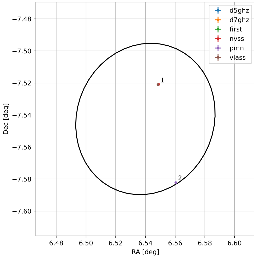
4FGL J0026.1-0732
