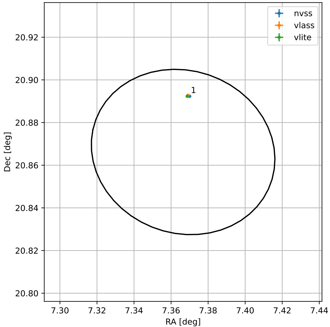
4FGL J0029.4+2051
