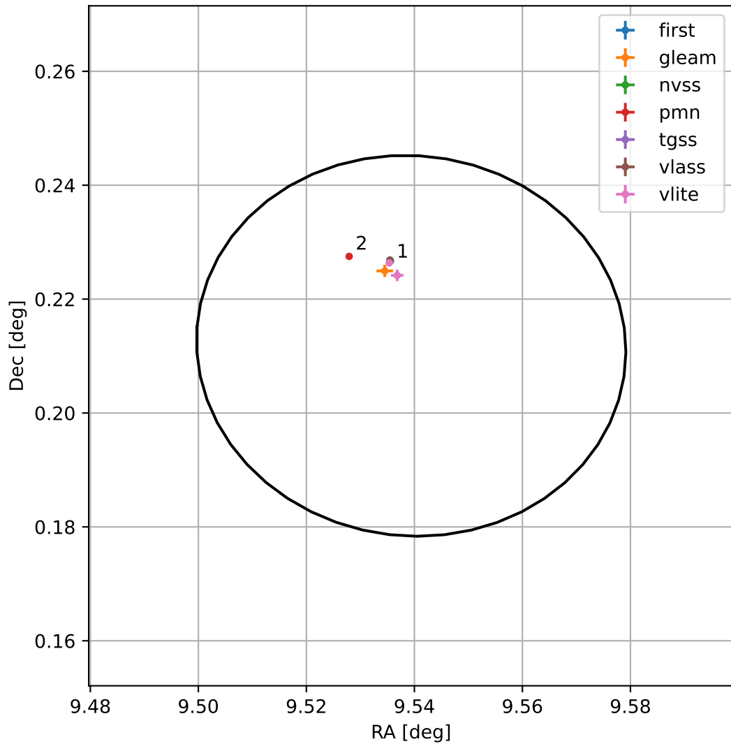
4FGL J0038.1+0012
