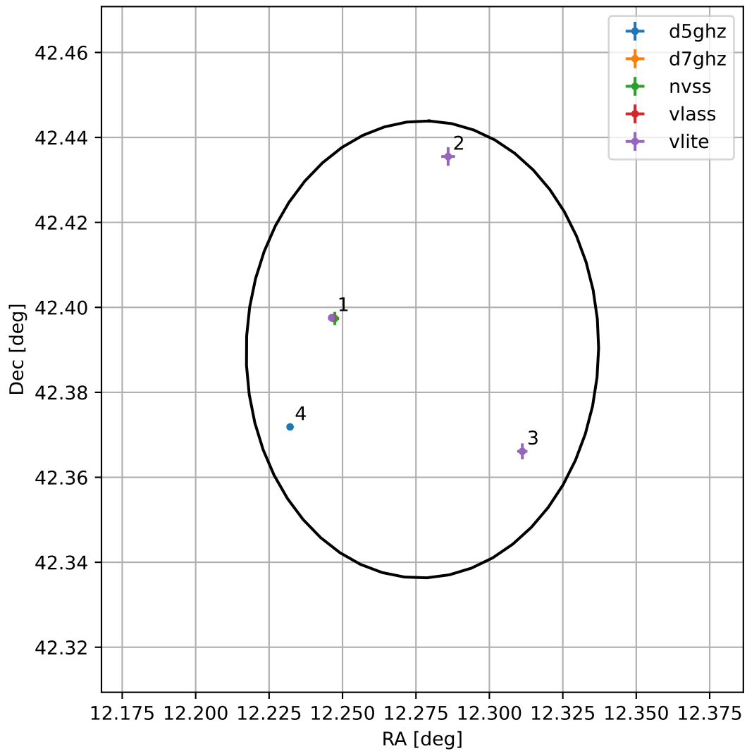
4FGL J0049.1+4223
