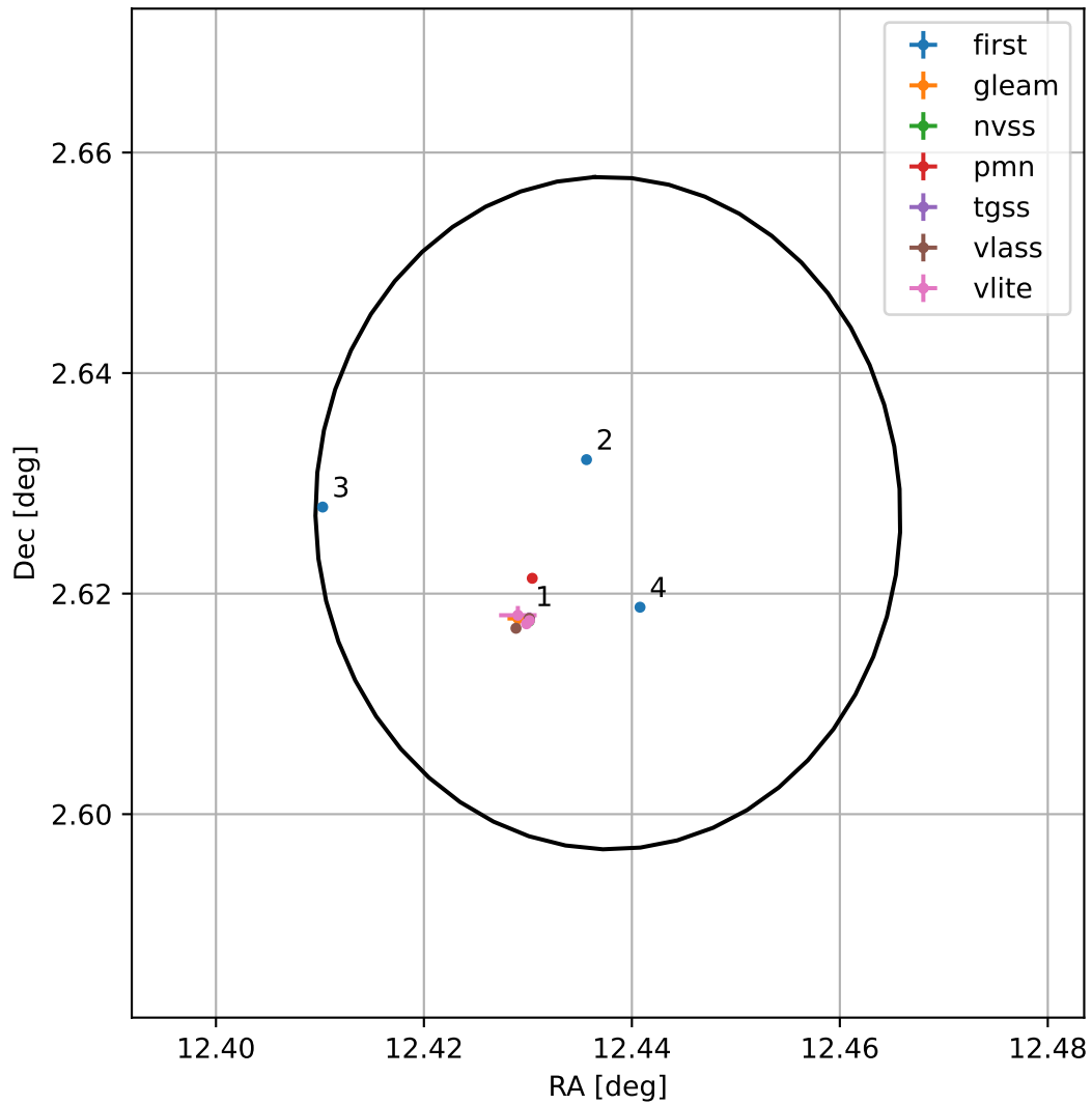
4FGL J0049.7+0237
