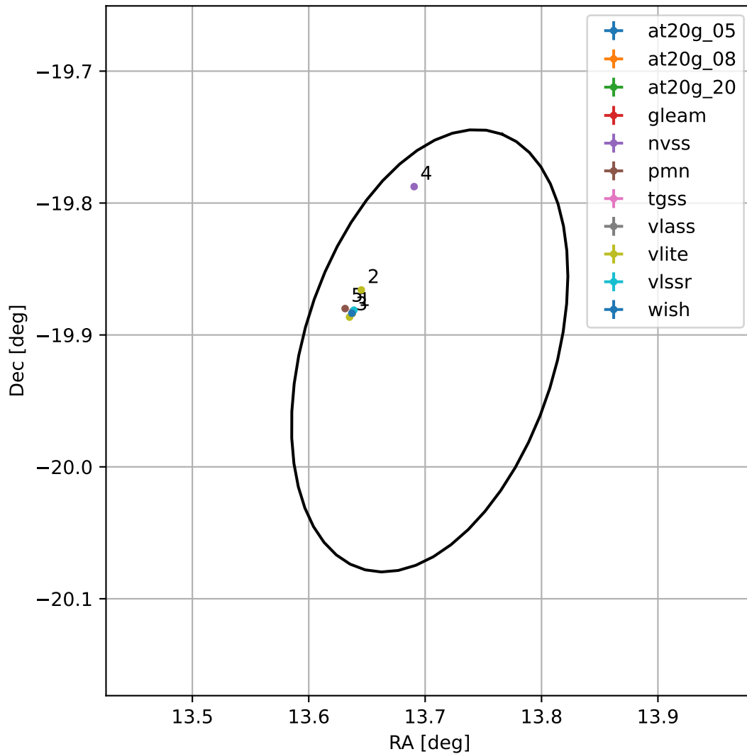
4FGL J0054.8-1954
