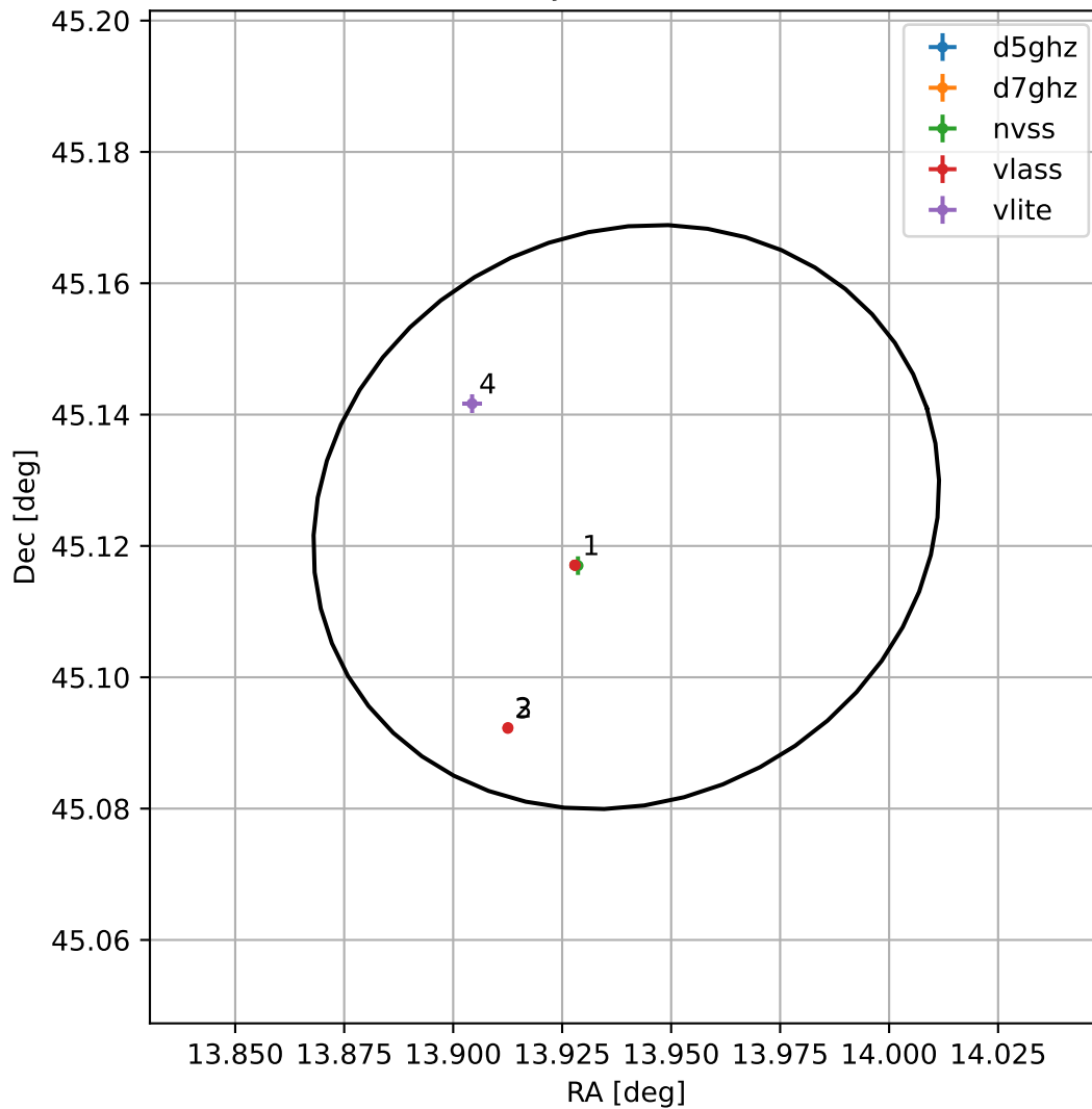
4FGL J0055.7+4507
