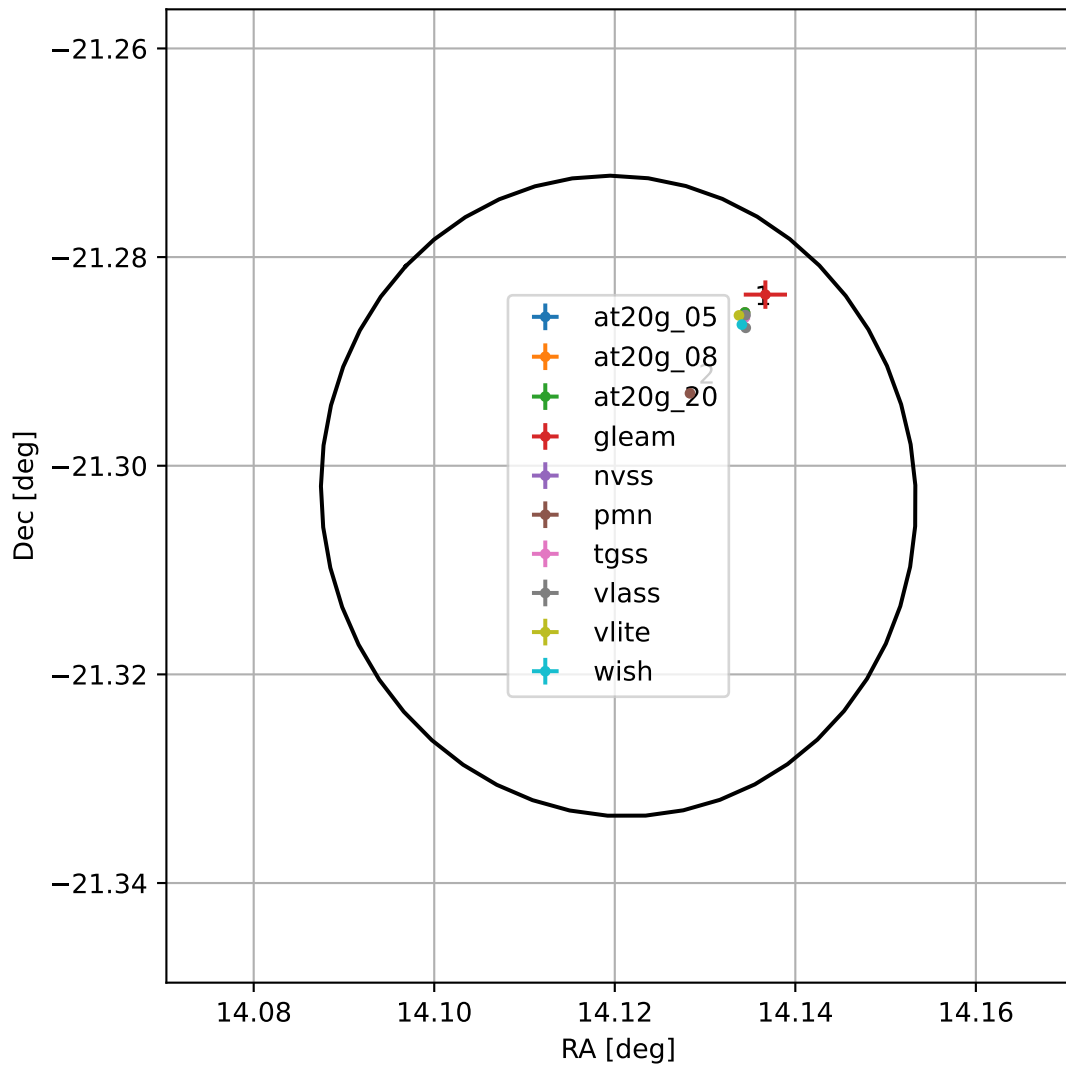
4FGL J0056.4-2118
