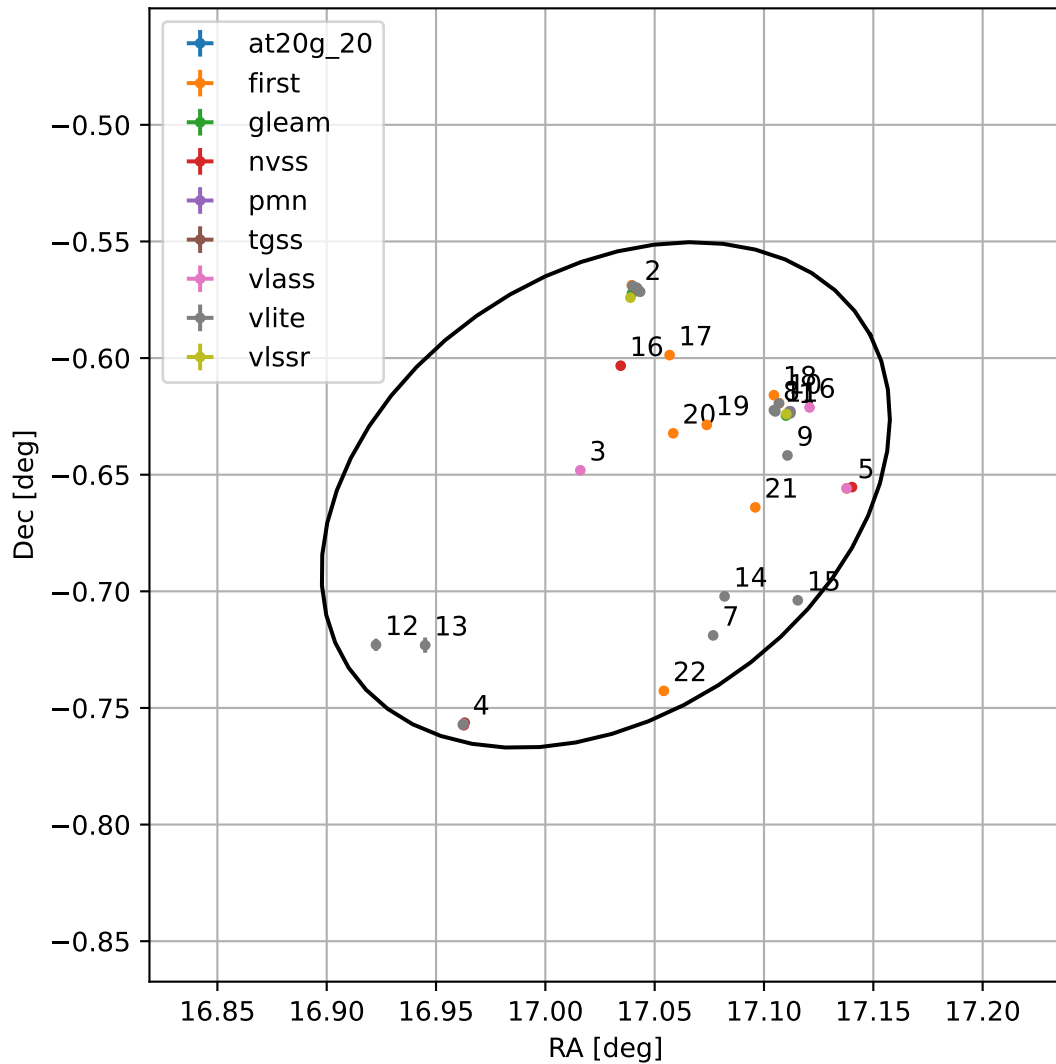
4FGL J0108.1-0039
