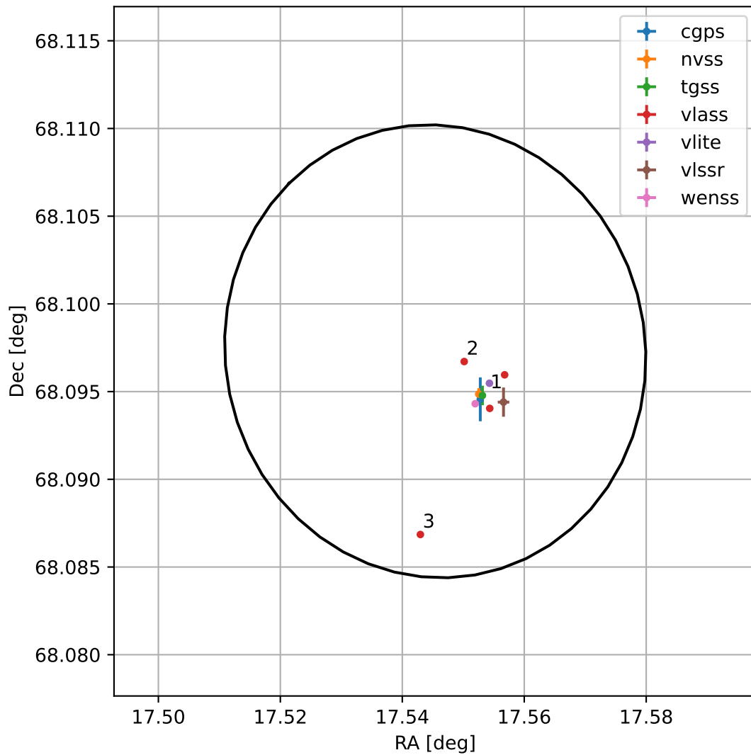
4FGL J0110.1+6805
