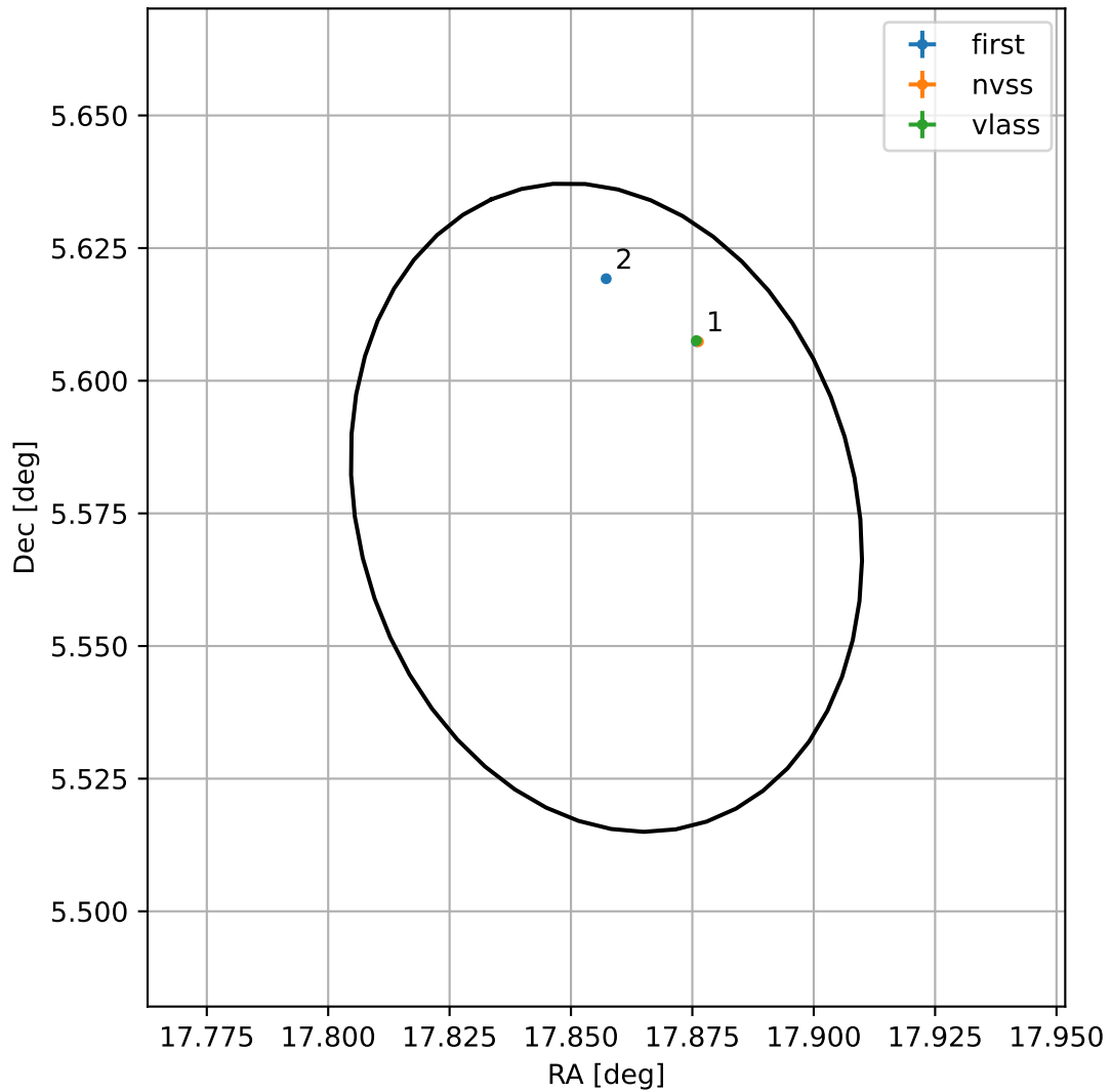
4FGL J0111.4+0534
