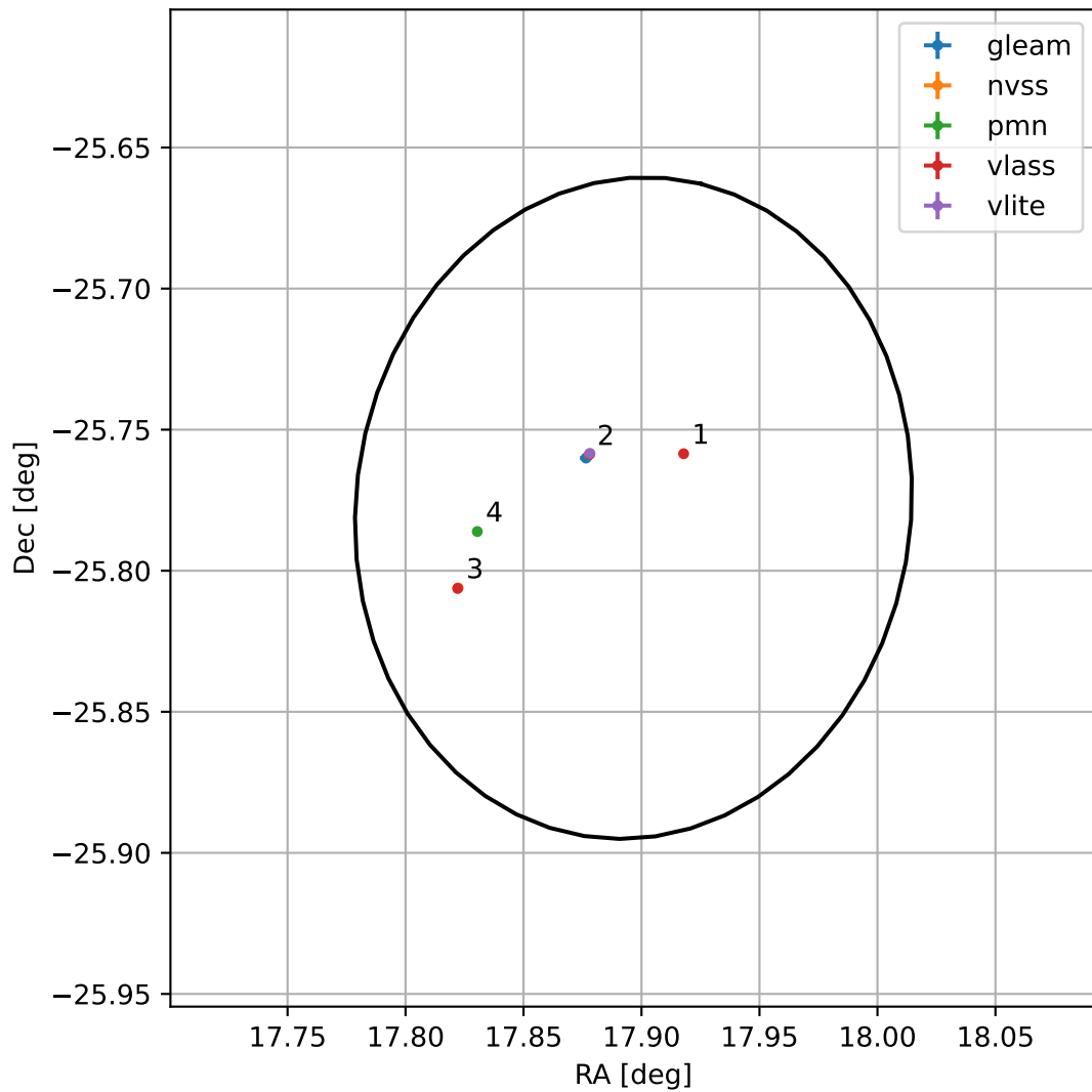
4FGL J0111.5-2546
