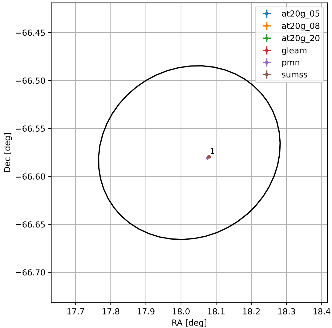
4FGL J0112.0-6634
