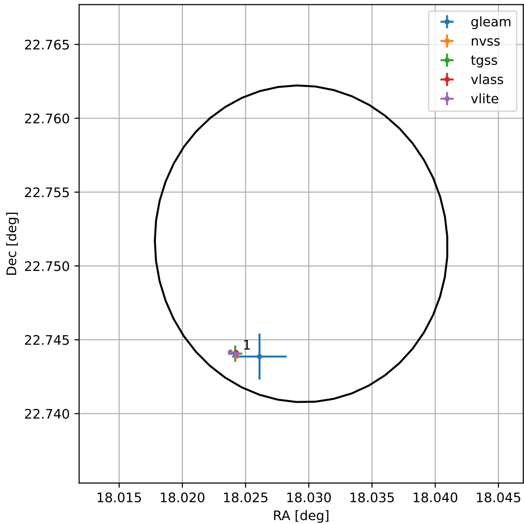
4FGL J0112.1+2245
