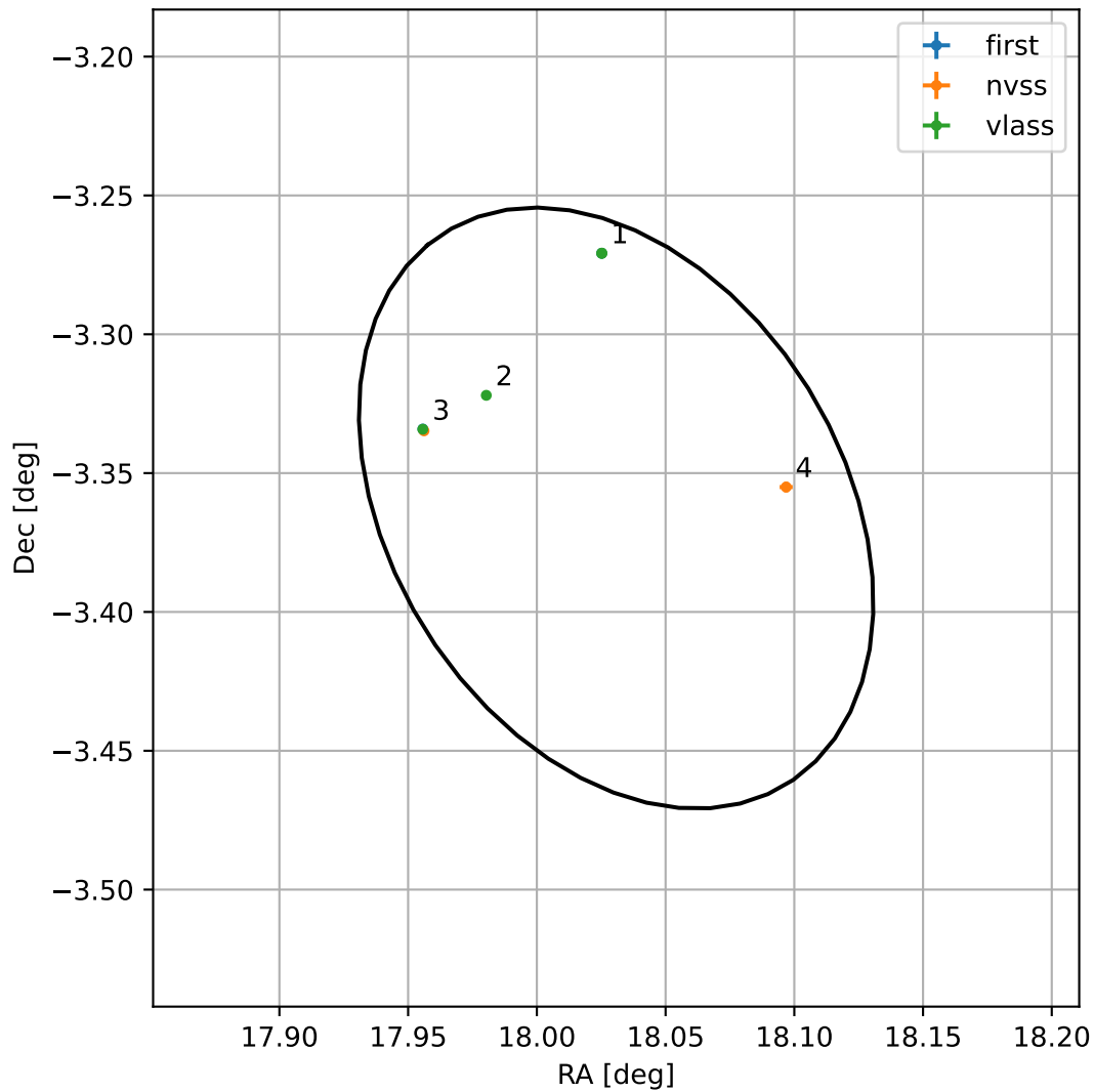
4FGL J0112.1-0321
