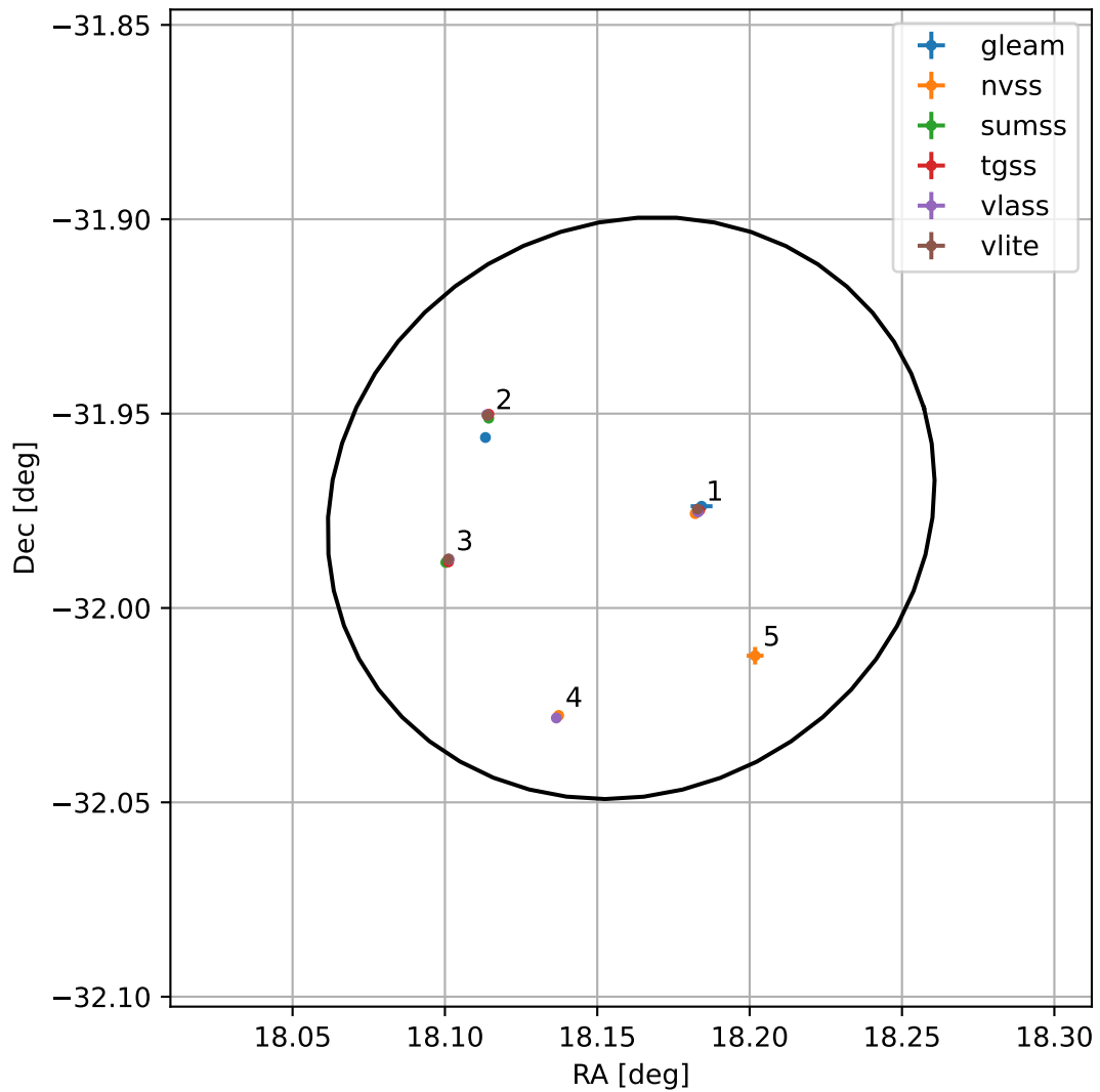
4FGL J0112.6-3158
