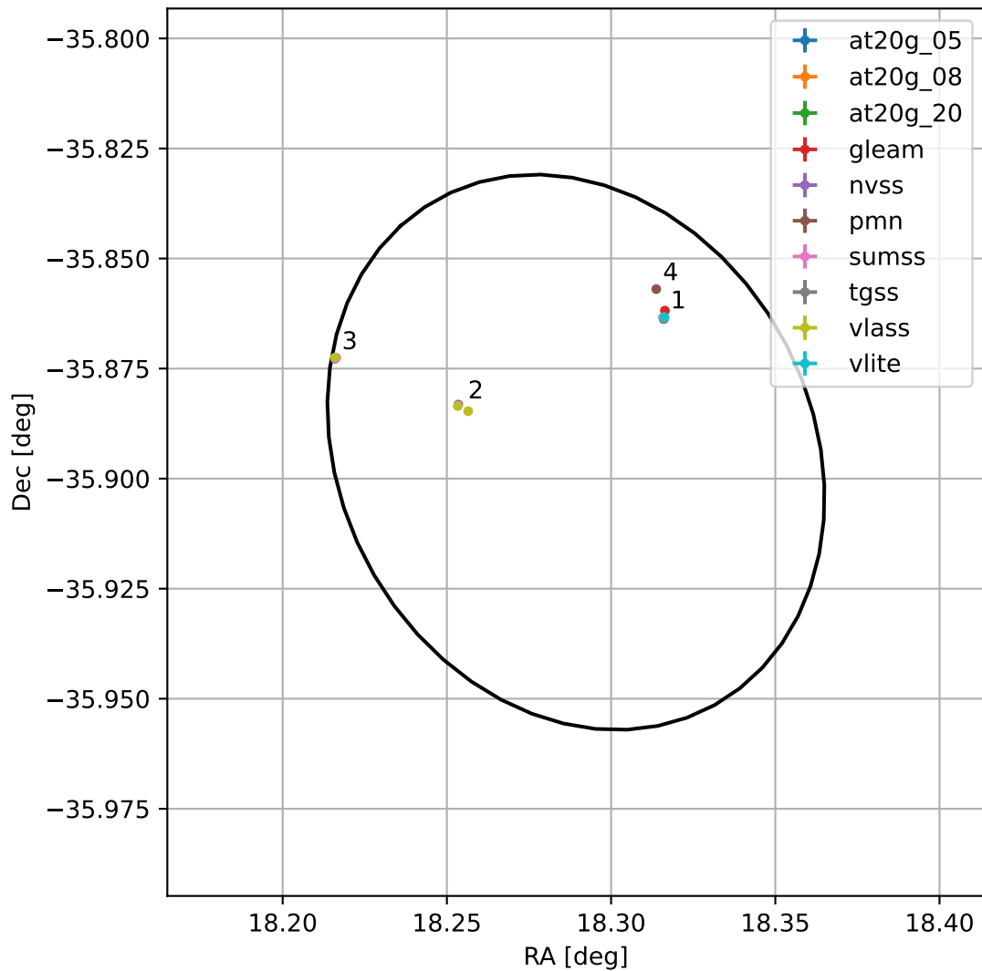
4FGL J0113.1-3553
