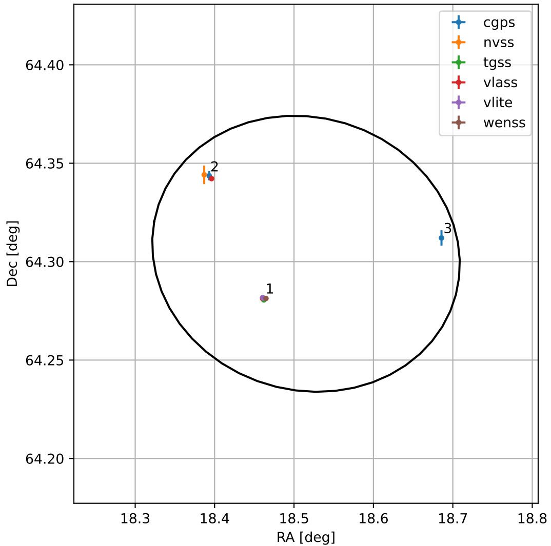
4FGL J0114.0+6418
