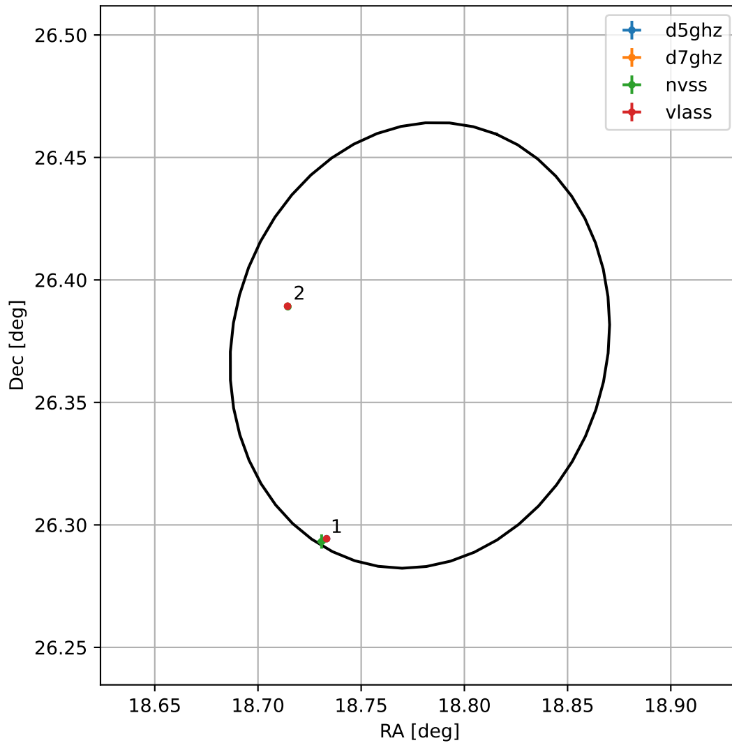
4FGL J0115.1+2622
