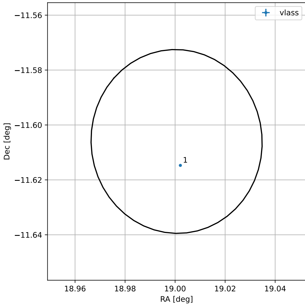
4FGL J0116.0-1136
