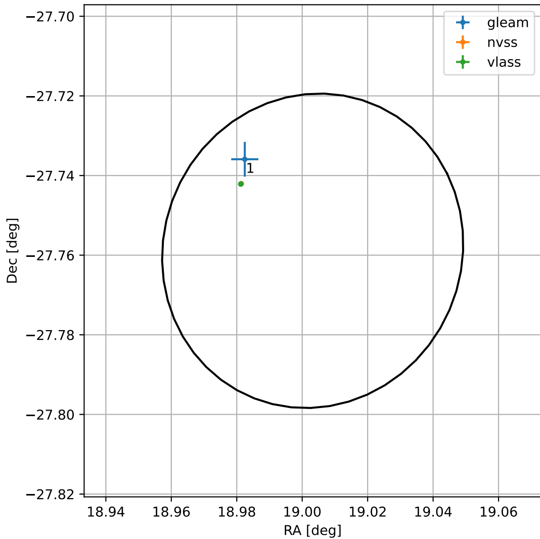
4FGL J0116.0-2745
