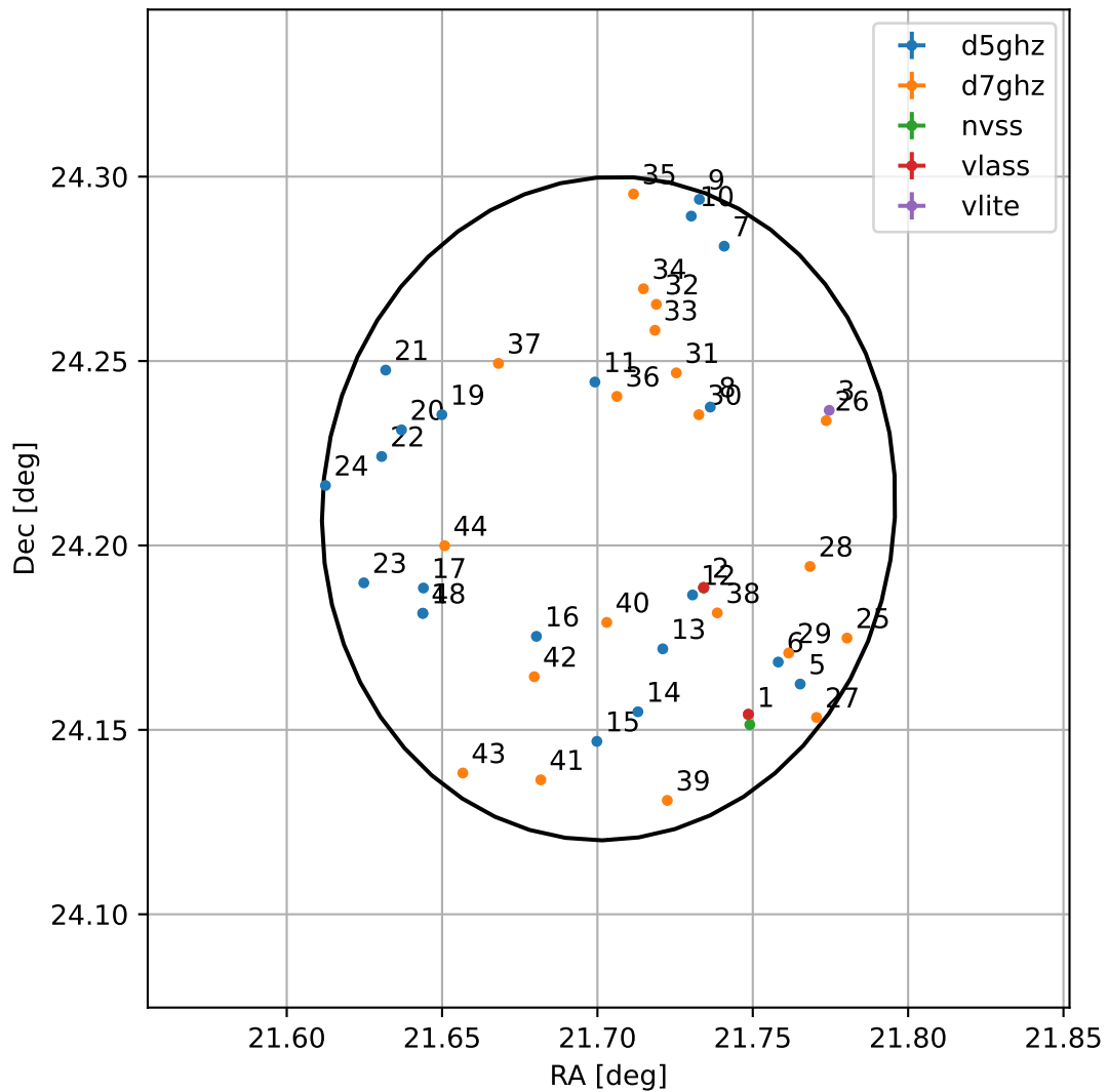
4FGL J0126.8+2412
