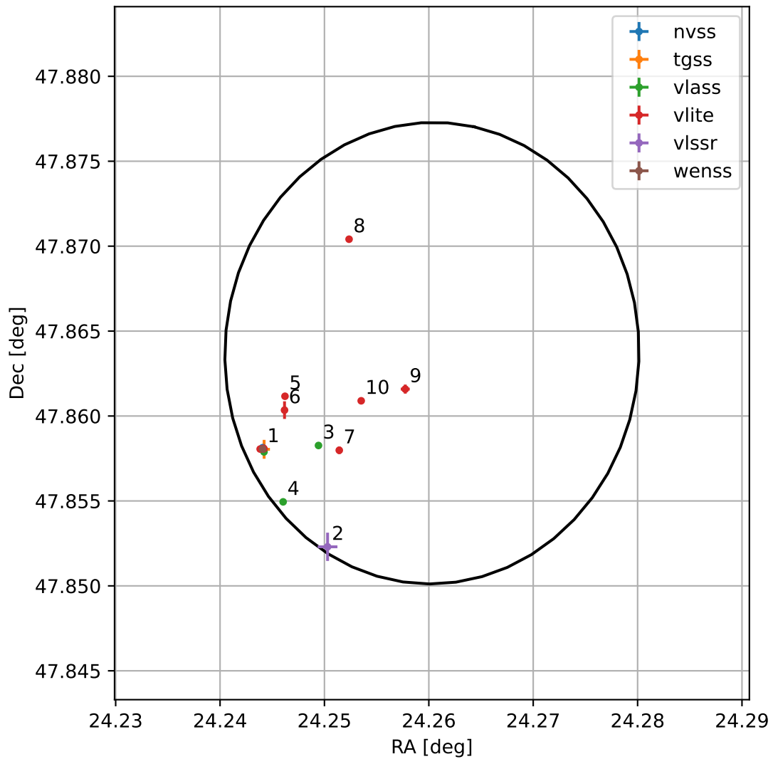
4FGL J0137.0+4751
