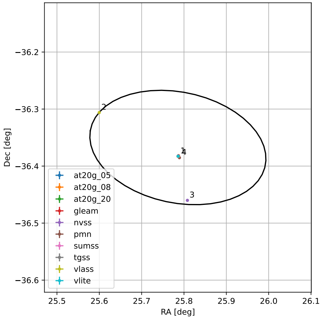
4FGL J0143.1-3622
