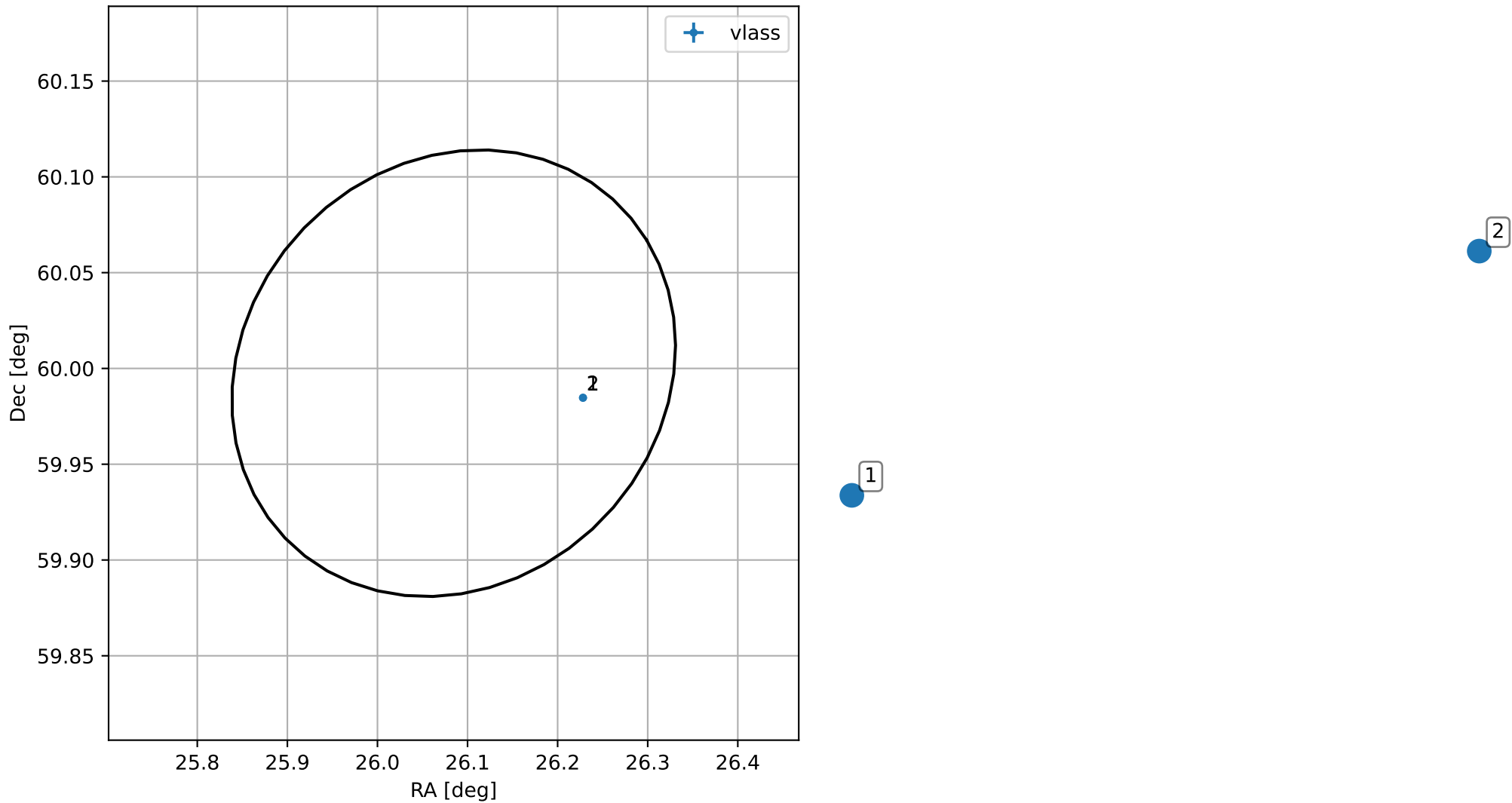
4FGL J0144.3+5959
