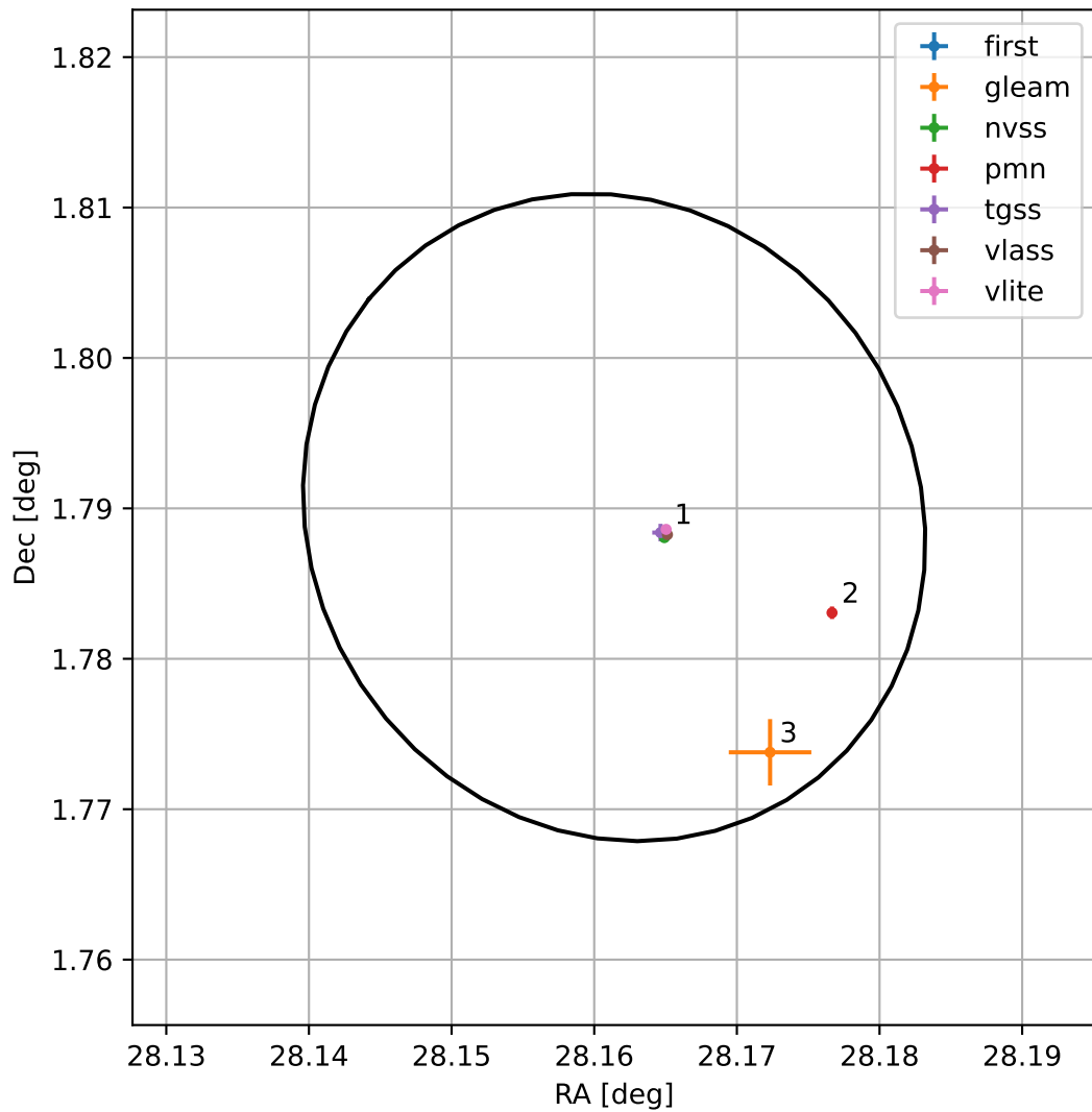
4FGL J0152.6+0147
