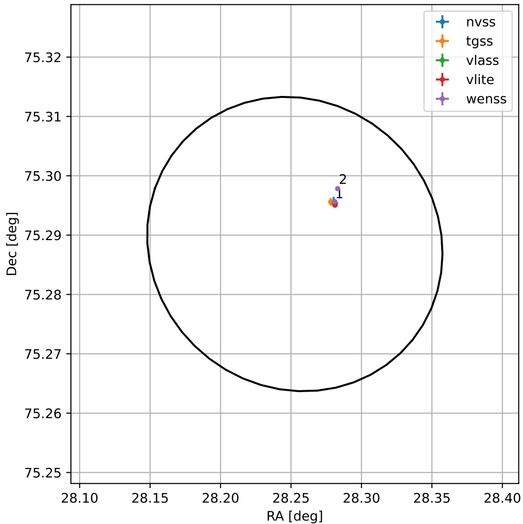
4FGL J0153.0+7517
