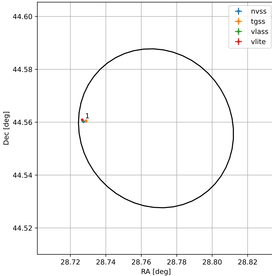
4FGL J0155.0+4433
