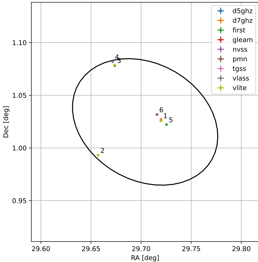
4FGL J0158.8+0101
