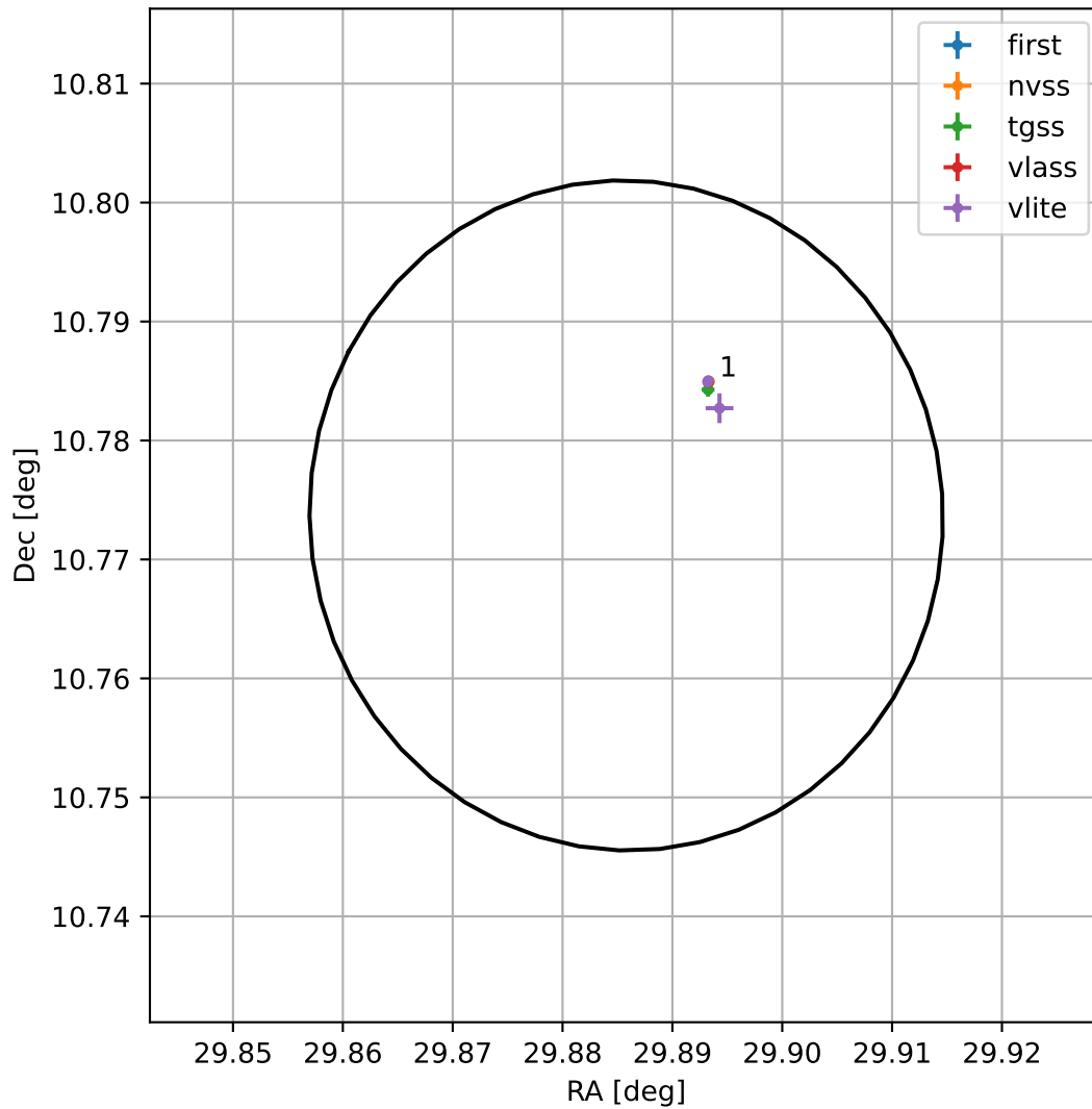
4FGL J0159.5+1046
