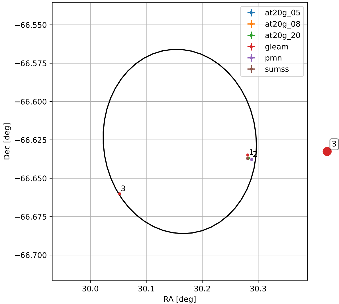
4FGL J0200.6-6637
