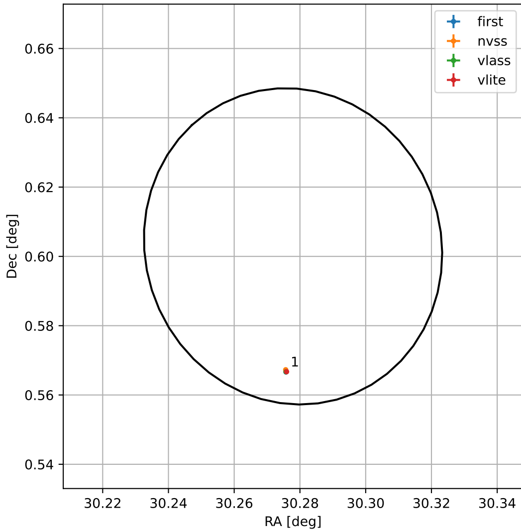
4FGL J0201.1+0036
