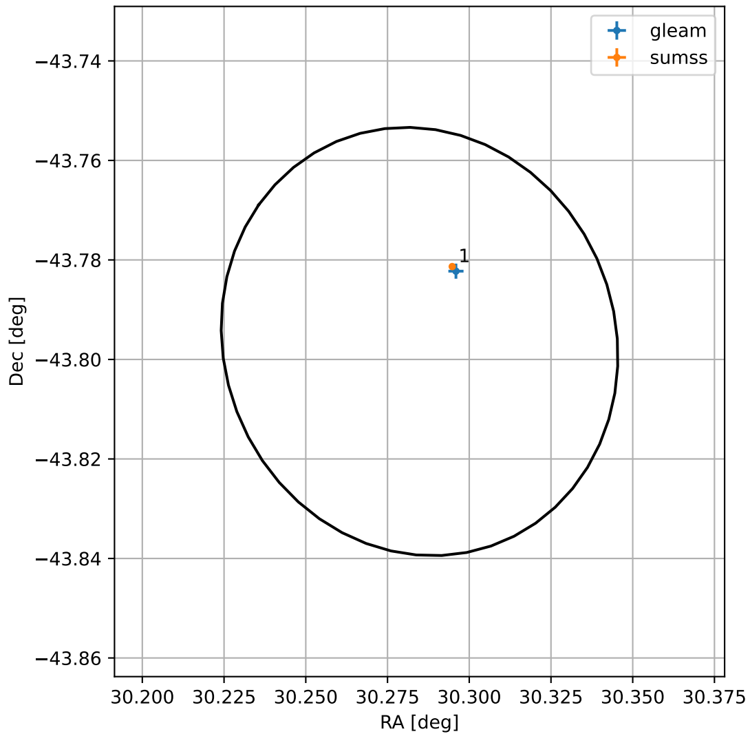
4FGL J0201.1-4347
