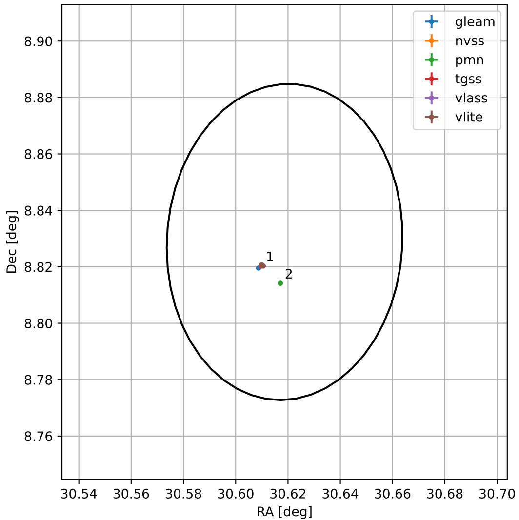
4FGL J0202.4+0849
