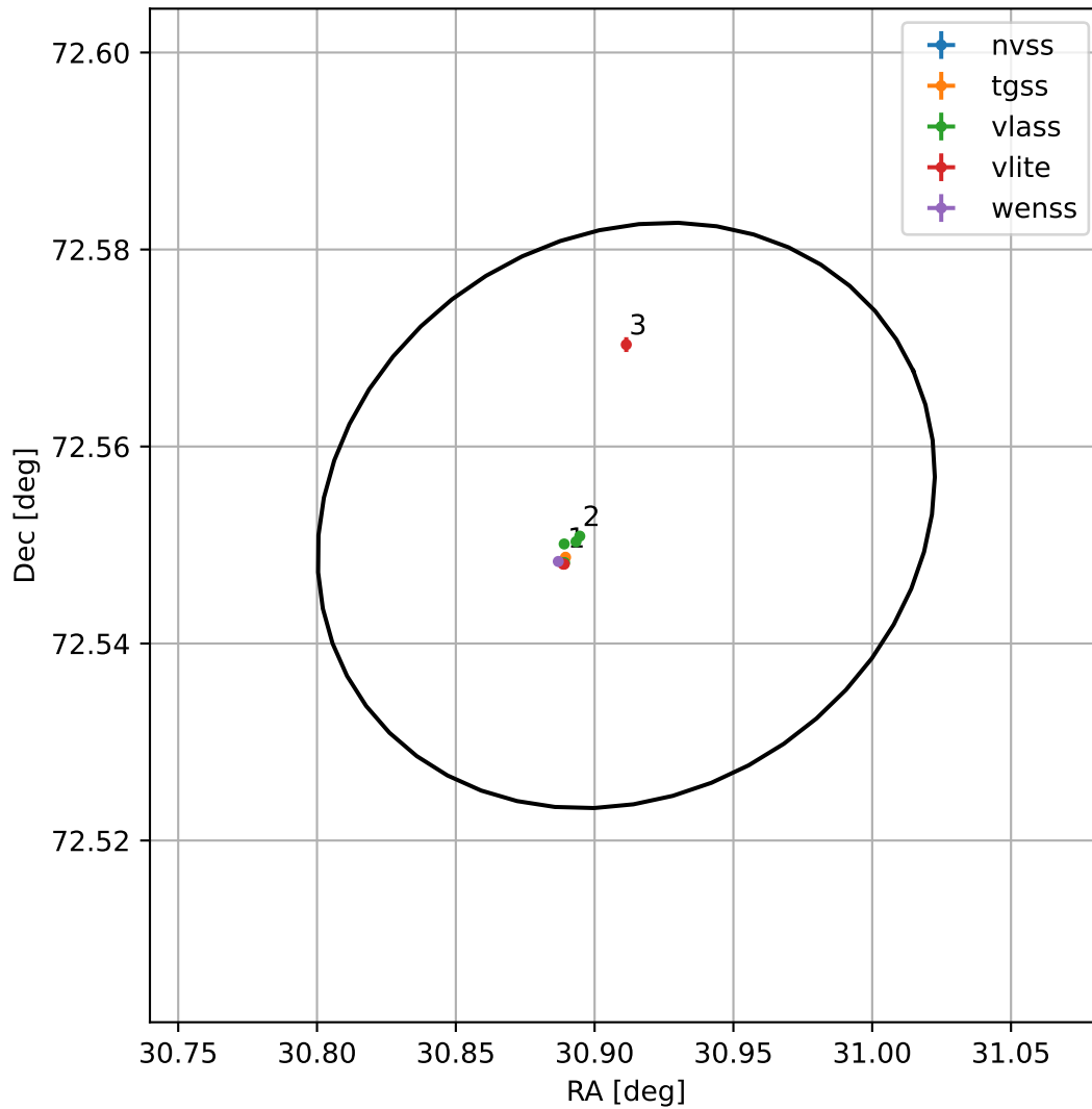
4FGL J0203.6+7233
