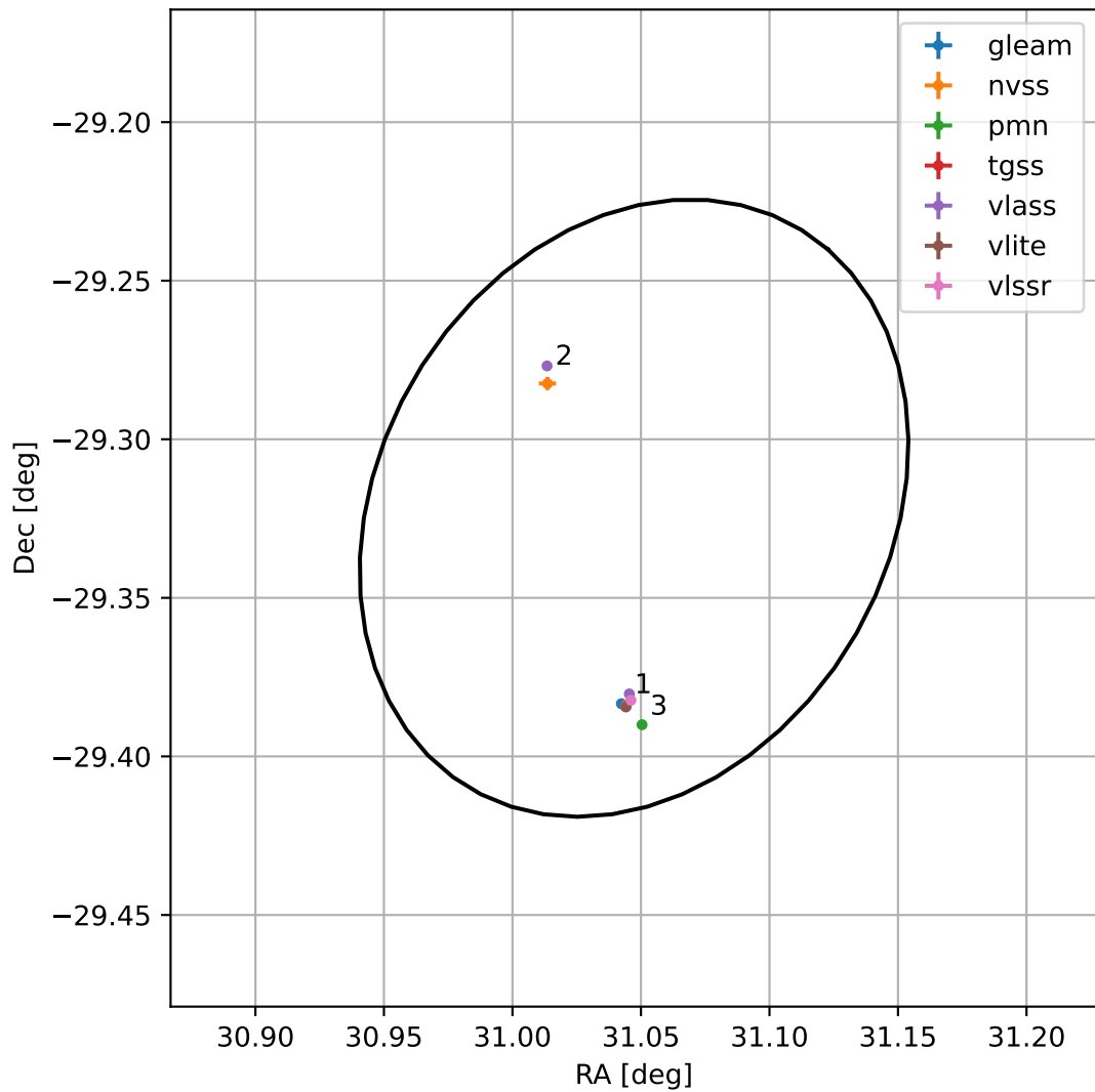
4FGL J0204.1-2919
