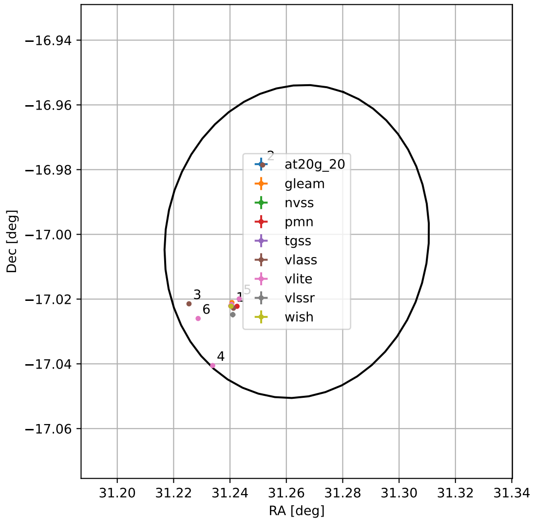
4FGL J0205.0-1700
